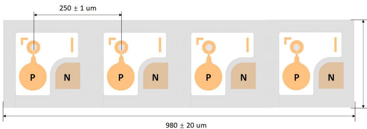
PN: QDV-294E (1x4 Array)
